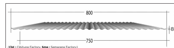
D-750 Thickness: Cbt : 20-30 Bj.L.S Smg : 20-30 Bj.L.S Minimum Length: Cbt : 1.50 m Smg : 1.50 m Maximum Length: Cbt : 1.829 m Smg : 3.658 m Spangle: Cbt : Min. Spangle Smg : With Spangle
